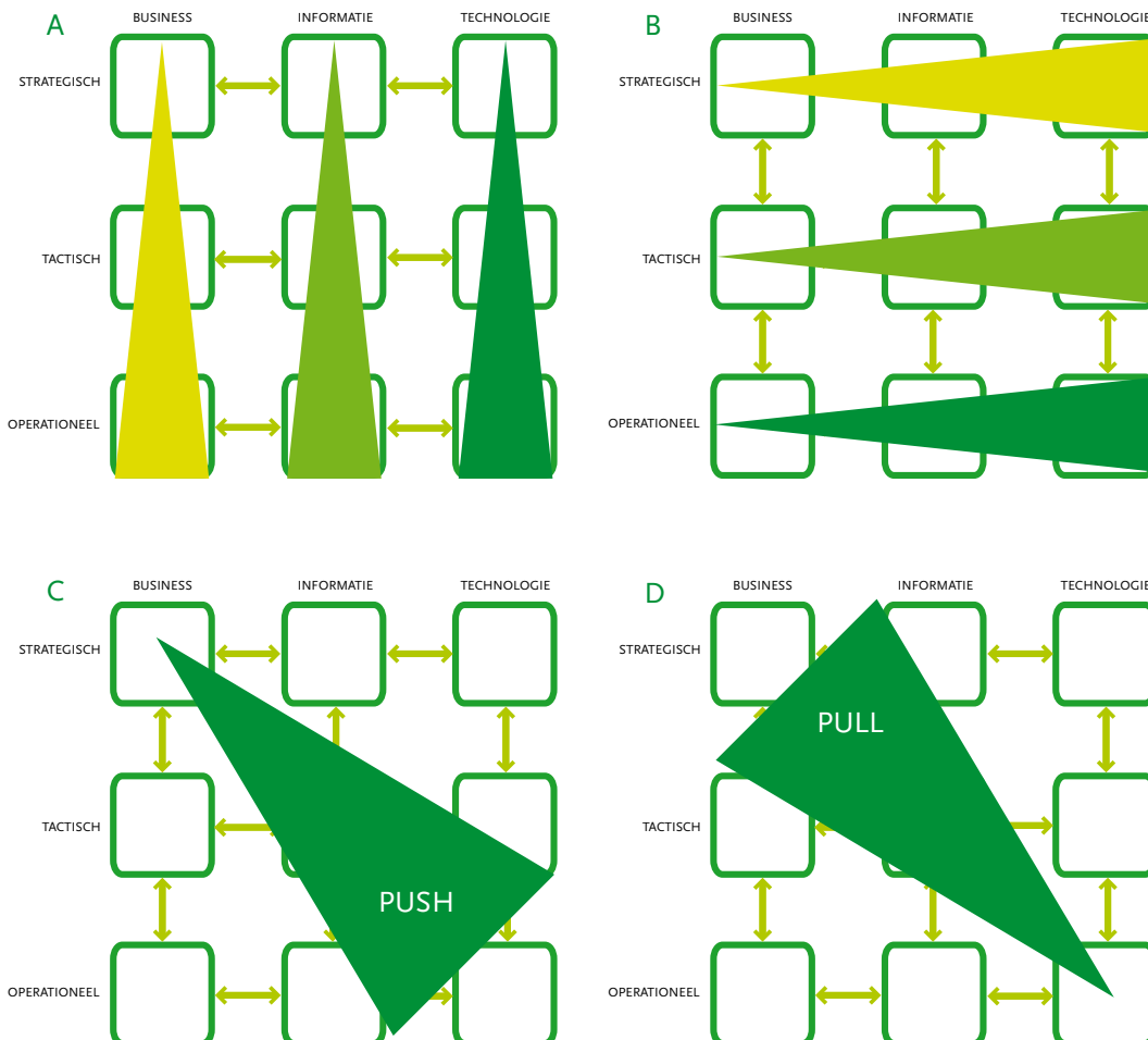
Figuur 16. Groei-scenario's
